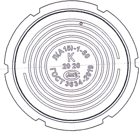
Люк чугунный тип Л для смотровых колодцев ГОСТ 3634-2019
